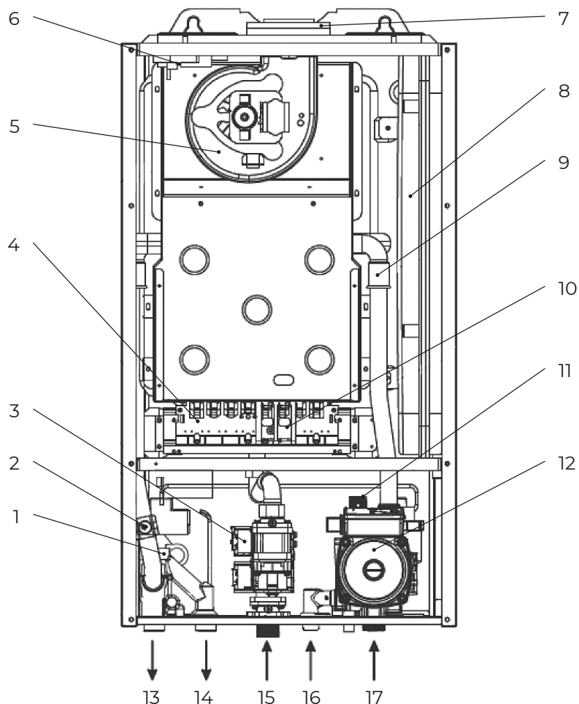
Рис. 4. Общая схема котлов В30 18 Н, 24 Н.
