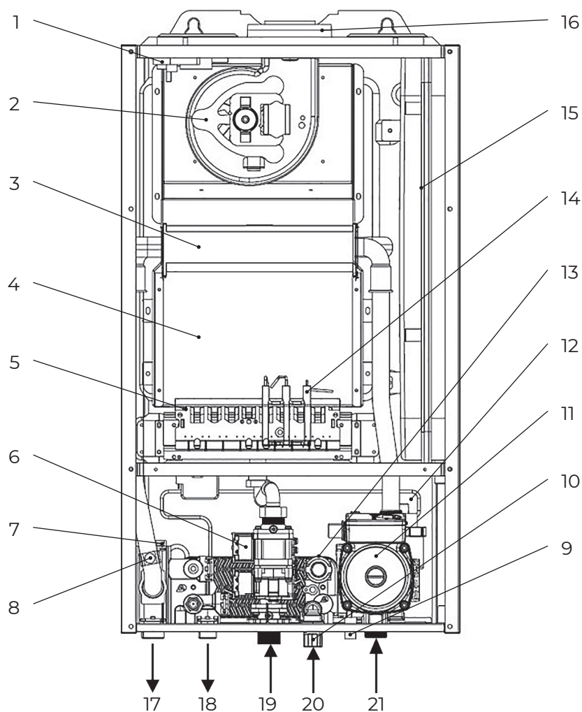
Рис. 2. Общая схема котлов B30 18 C, 24 C.
