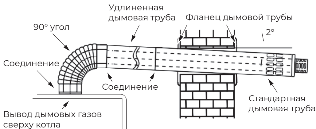
Рис. 30. Пример монтажа схемы С12.
