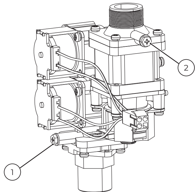
Рис. 25. Газовый клапан.
