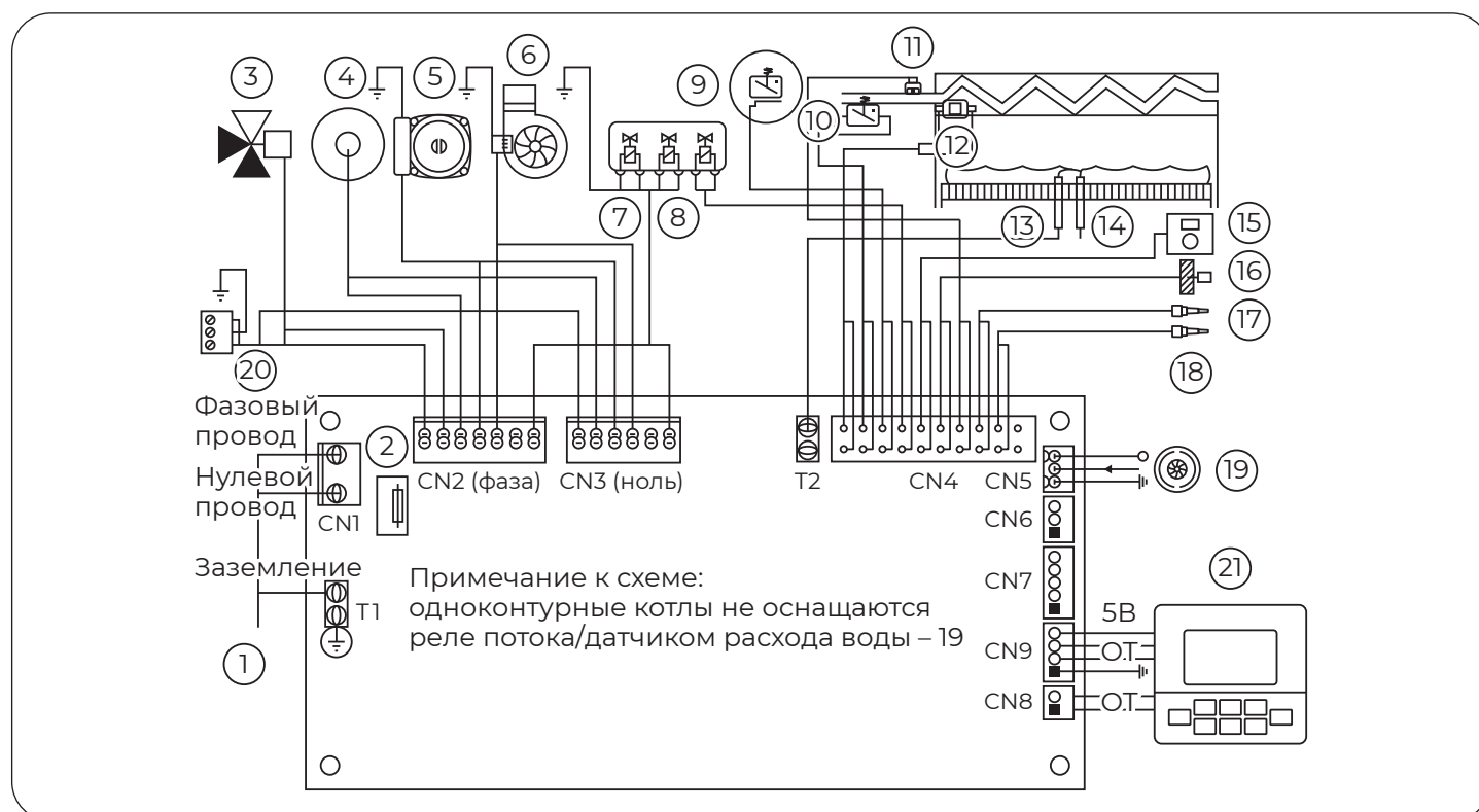
Рис. 31. Электрическая схема.
