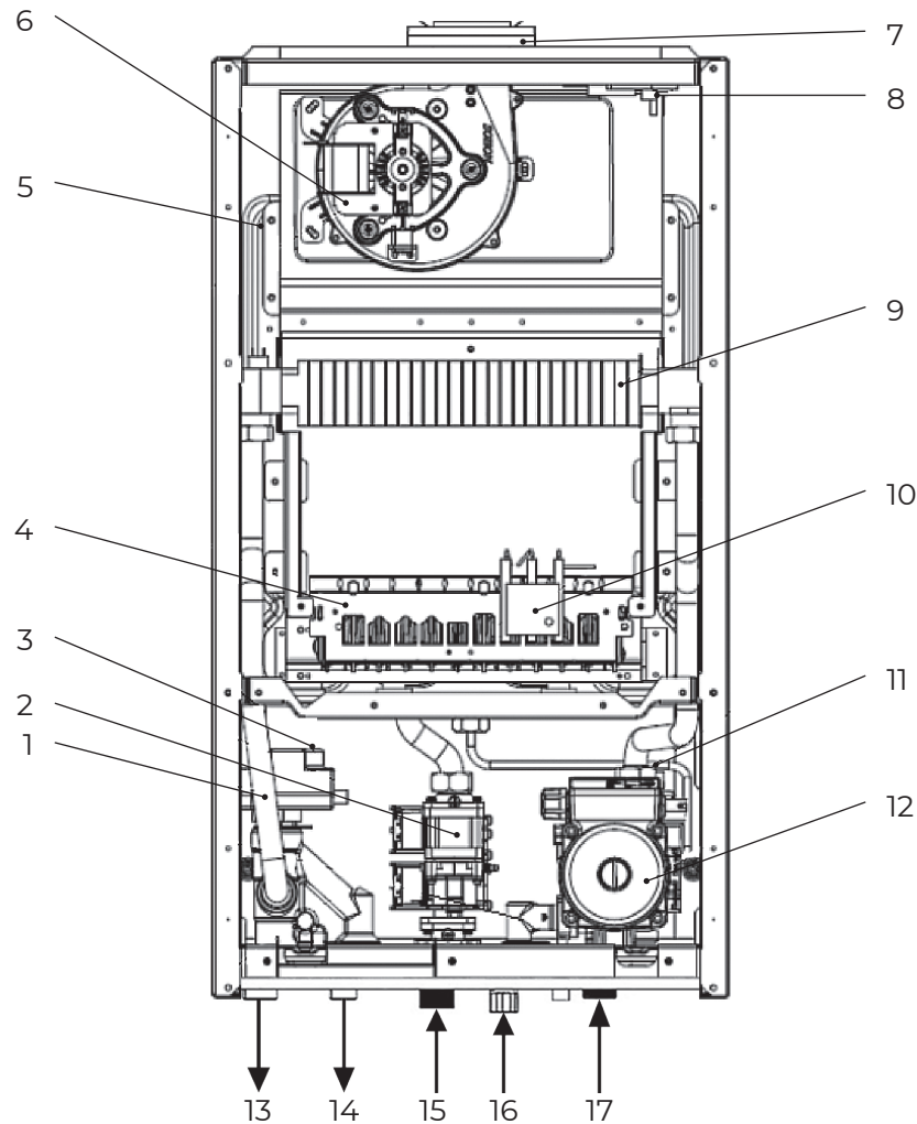
Рис. 5. Общая схема котлов B30 28 H, 32 H, 36 H.
