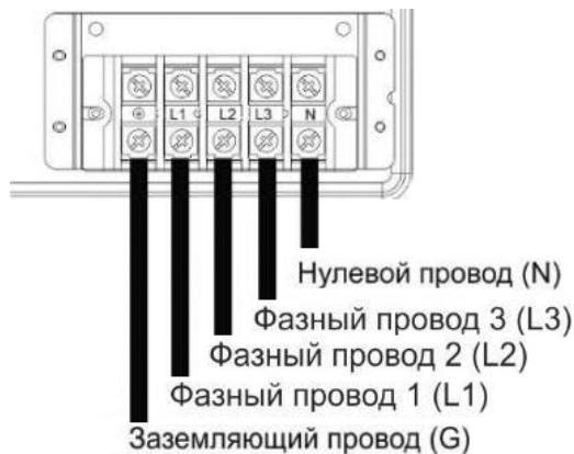
Рис 11. Трехфазное подключение прибора
