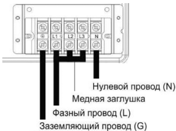
Рис 10. Однофазное подключение прибора
