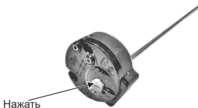
Рис.2. Расположение штока на термовыключателе термостата
