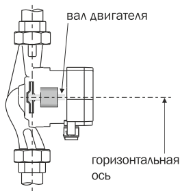
Правильная установка насоса на вертикальном участке трубопровода
